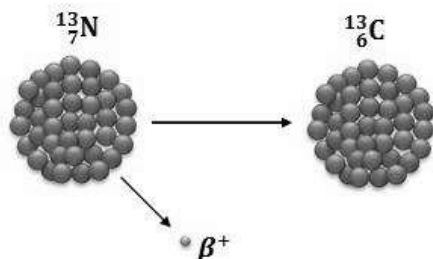
Slika 9. Raspad N-13
