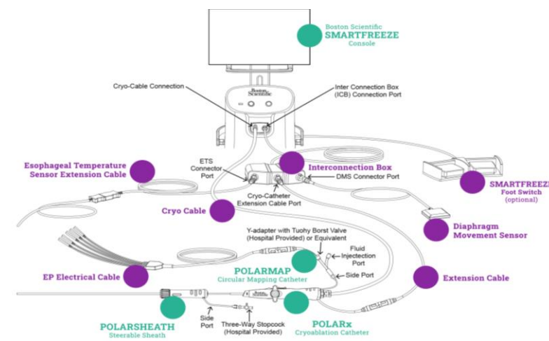
Slika 8. Ilustrirani prikaz sustava i opreme potrebne za krioablaciju (izvor https://www.educare-singleshot.eu/ ).
