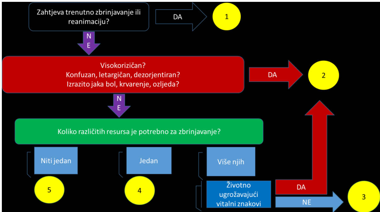
Slika 2 ESI algoritam
